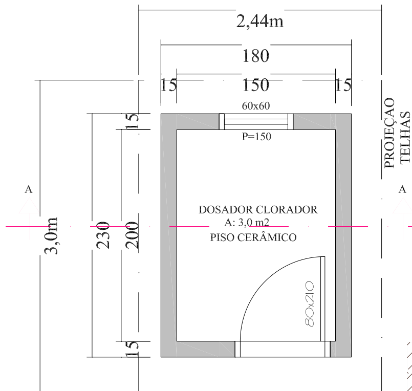
PLANTA BAIXA CORTE A-B ESC. 1:50
